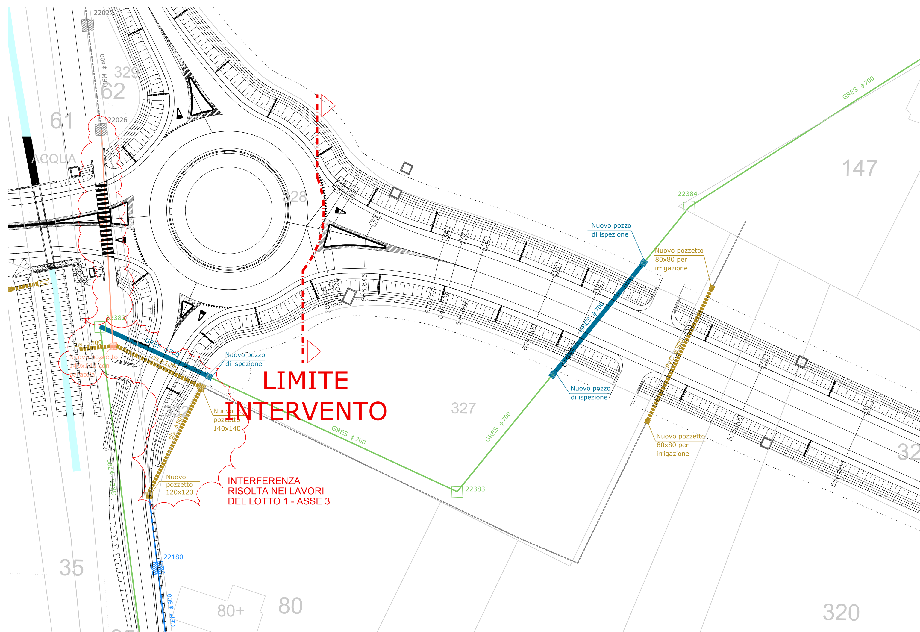
PARTICOLARE A - Progetto - SCALA 1:500
