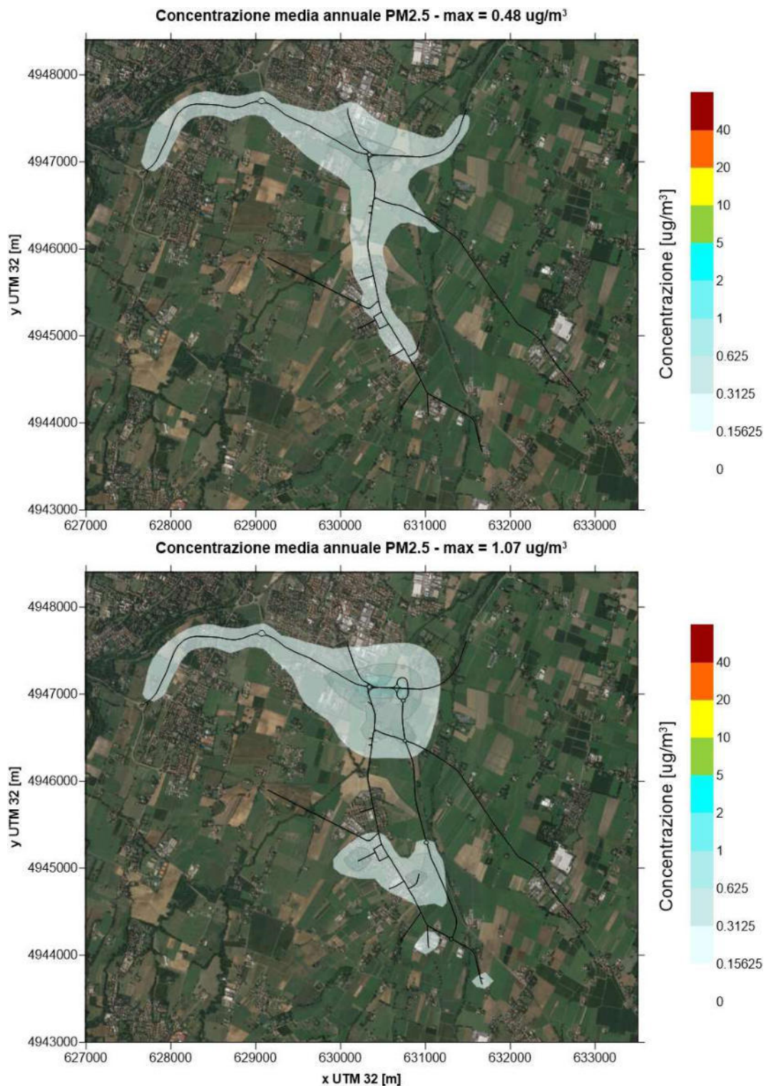
Figura 10. Media annuale delle concentrazioni giornaliere di PM 2.5 [µg/m 3 ] nello scenario base (sopra) e in quello futuro (sotto)
