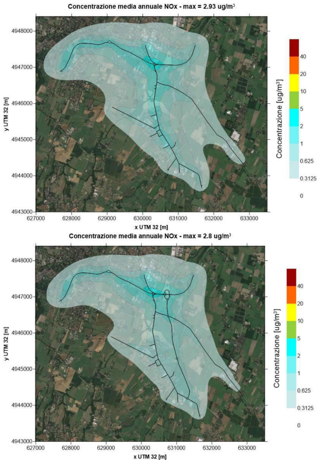
Figura 8. Media annuale delle concentrazioni medie orarie di NO 2 [µg/m 3 ] nello scenario base (sopra) e in quello futuro (sotto)
