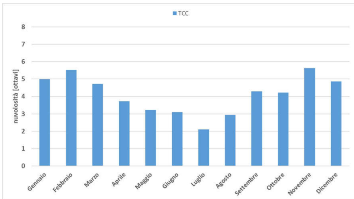
Figura 4. Nuvolosità media mensile per l'intero periodo di simulazione.
