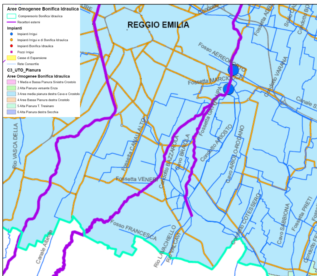
Figura 2.2 – Estratto "Aree omogenee di bonifica idraulica" – Piano di Classifica del Consorzio di Bonifica dell'Emilia Centrale
