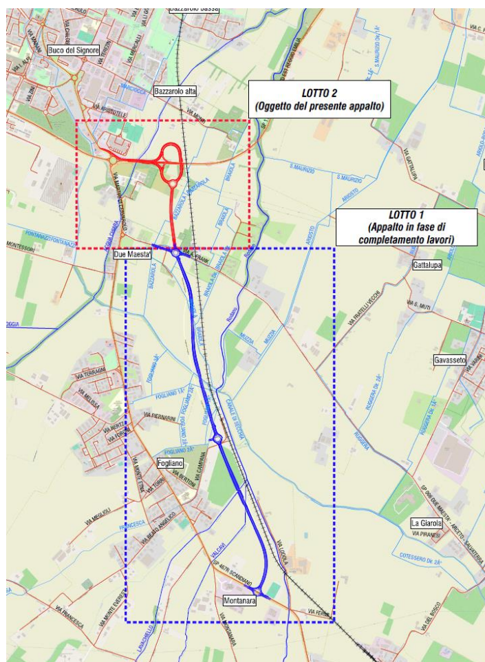
Figura 2.1 – Corografia generale del reticolo idrografico presente nell'area di intervento
