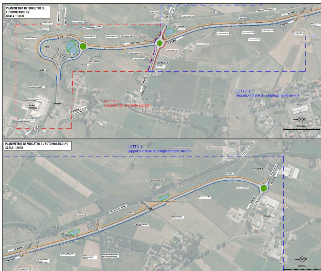
Figura 4.1 – Inquadramento del progetto
