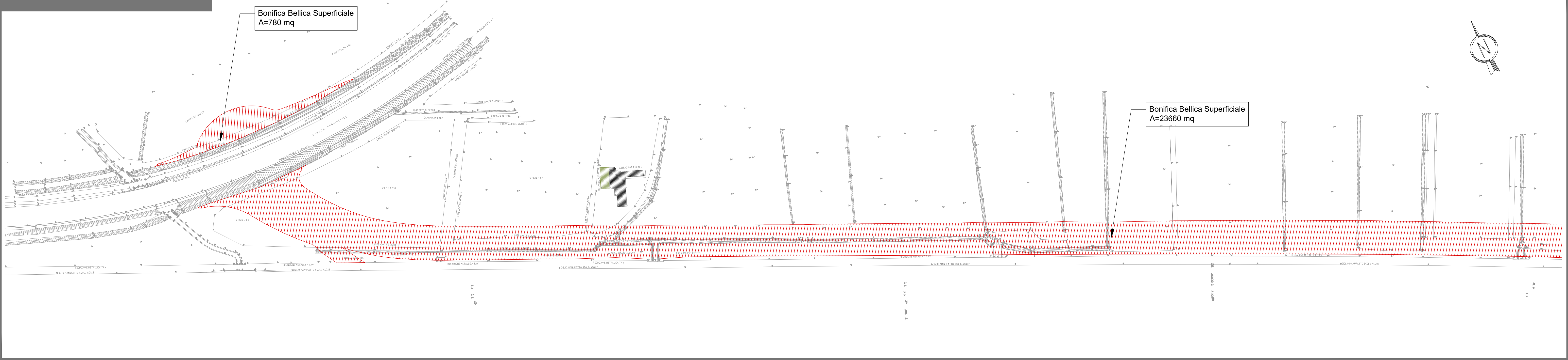
PLANIMETRIA RIQUADRO 1 - scala 1:1000
