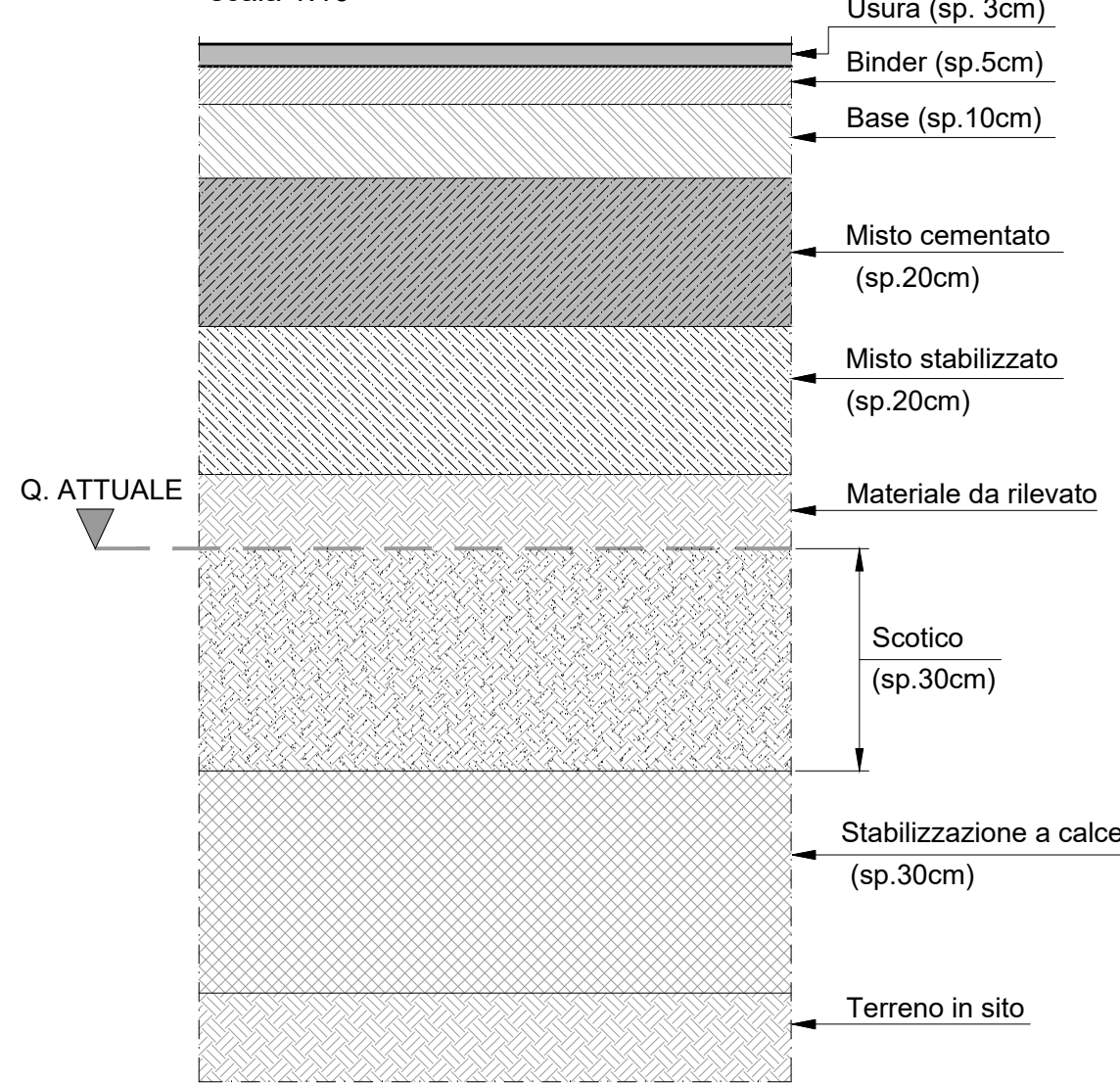
PACCHETTO A - STRADALE scala 1:10
