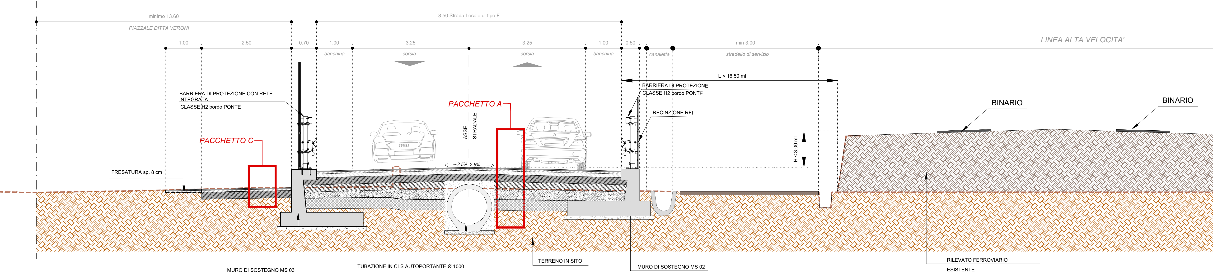
DEMOLIZIONI RETI "DITTA VERONI" scala 1:1000
