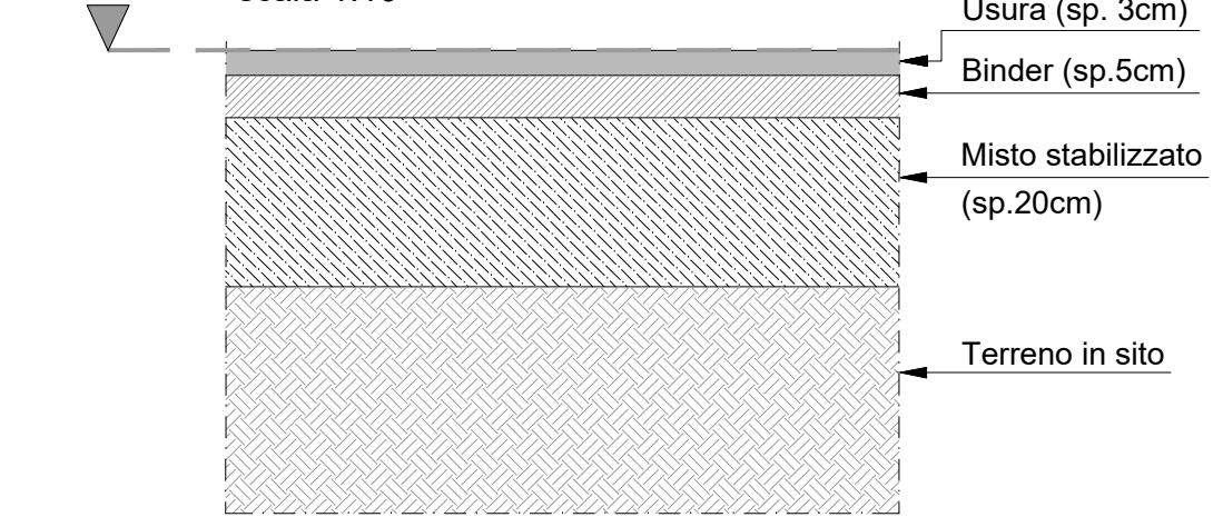
PACCHETTO C - PIAZZALE "DITTA VERONI" scala 1:10
